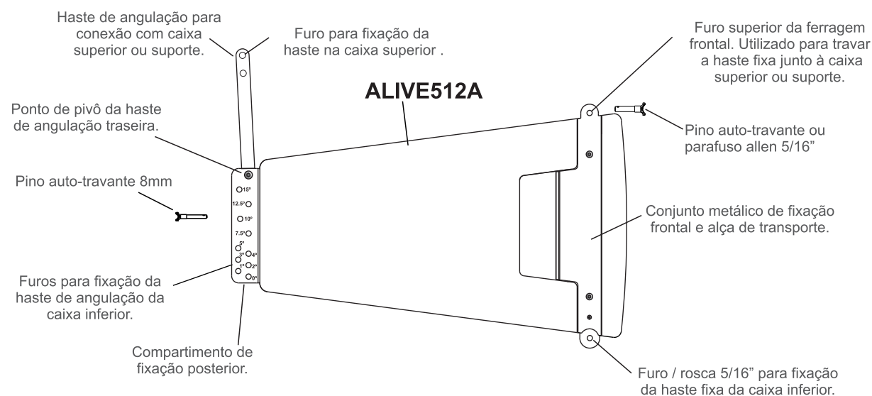
Figura 2 - Caixa-acústica Série ALIVE.
